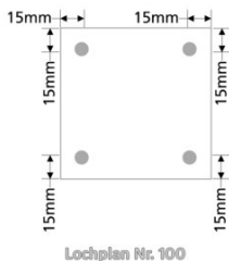
Lochplan Nr. 100
